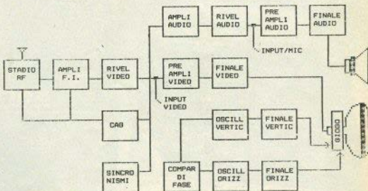
fig. 1: schema essenziale di un televisore.
